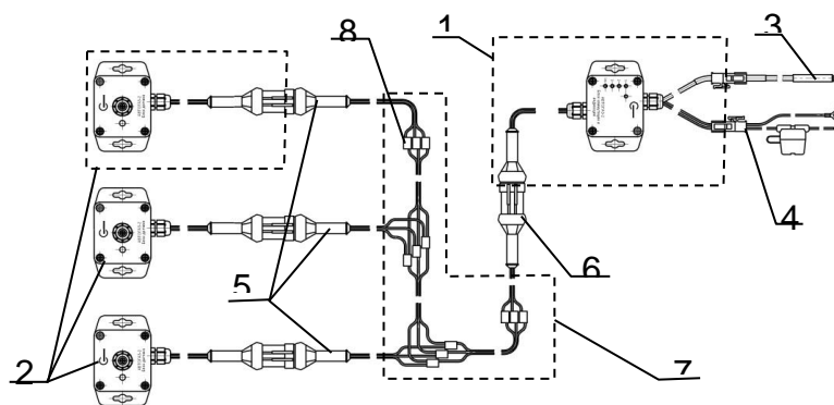
Рисунок 2 – Схема соединений блоков Системы
